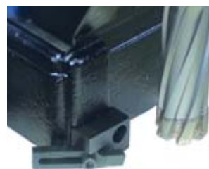
Насадка для дробления стружки
